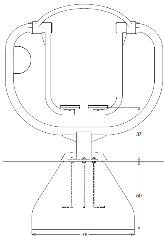
Plan de fundație (vedere față) — montaj prin încadrare directă pe placă de beton existentă
