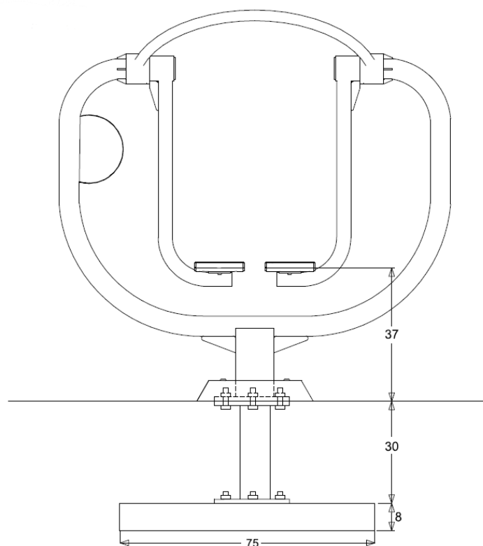
Plan de fundație (vedere față) — montaj în fundație de beton, timp întărire min. 48 ore
