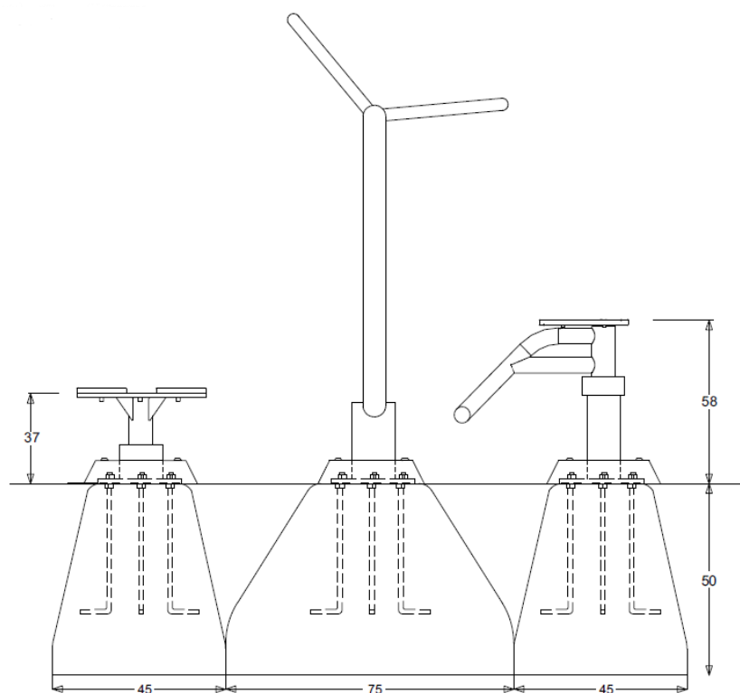
Plan de fundație (vedere față) — montaj prin încadrare directă pe placă de beton existentă
