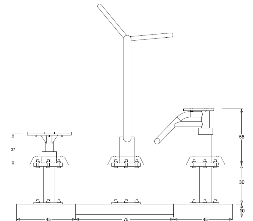
Plan de fundație (vedere față) — montaj în fundație de beton, timp întărire min. 48 ore
